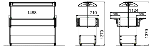
KORO 4/1 Caldo (Baino Maria) - Hot (Bain Marie) Heiß (Bain Marie) - Chaud (Bain Marie) - Caliente (Baino Maria)
