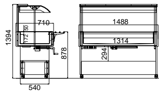
KORO 4/1 MURALE Refrigerato - Cold - Refrigeré - Kalt - Refrigerado
