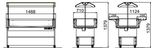
KORO 4/1 Refrigerato - Cold - Kalt - Réfrigéré - Refrigerado
