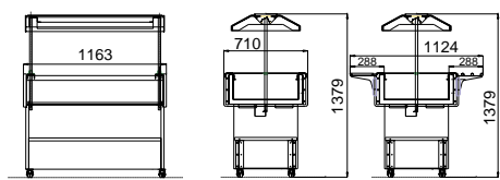
KORO 3/1 Refrigerato - Cold - Kalt - Réfrigéré - Refrigerado
