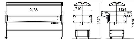
KORO 6/1 Refrigerato - Cold - Kalt - Réfrigéré - Refrigerado
