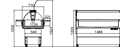
KORO WINGS Refrigerato - Cold - Kalt - Réfrigéré - Refrigerado
